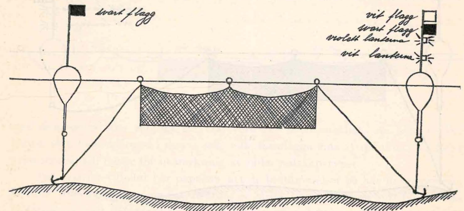
Utmärkning av redskap förankrad i båda ändar.
